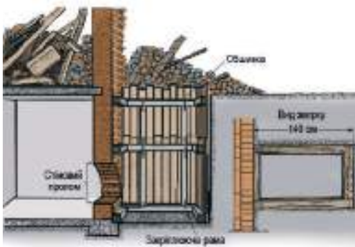
Іл. 34.11. Шахта
