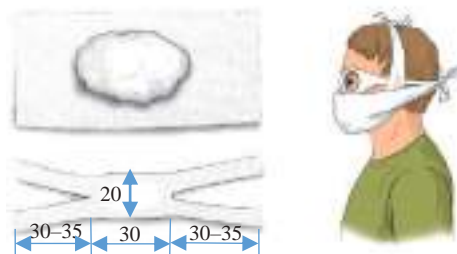
Іл. 27.5. Виготовлення ватно-марлевої пов'язки (розміри у см)
