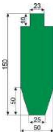
Іл. 1.10. Мішень № 8 — лінійні розміри у см
